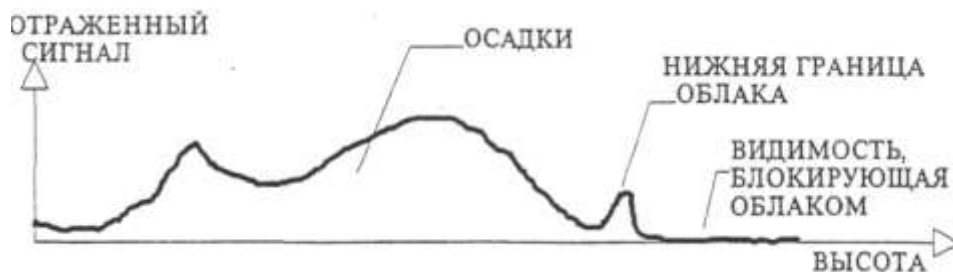
Рис.1 Типичный сигнал измерения
